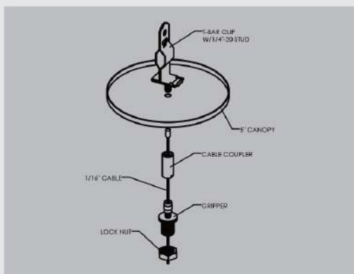
Option de montage sur plafond en T
