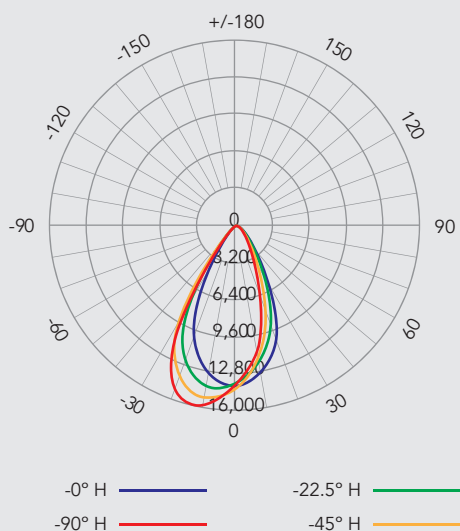
RÉPARTITION ANGULAIRE DE L'INTENSITÉ (BANDE DE 2,4 M [8 PI])
