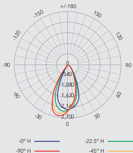
RÉPARTITION ANGULAIRE DE L'INTENSITÉ (BANDE DE 0,6 M [2 PI])
