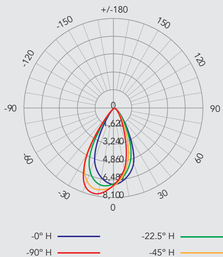
RÉPARTITION ANGULAIRE DE L'INTENSITÉ (BANDE DE 1,2 M [4 PI])
