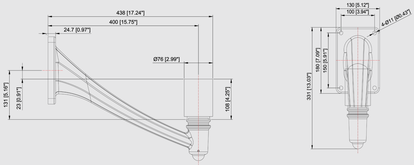
R59025 - Arm
