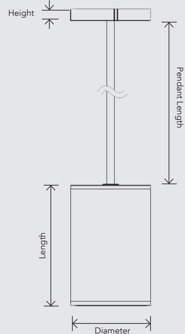
Pendant Mount
